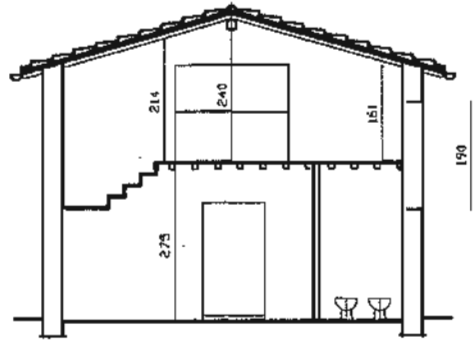
SEZIONE X-X invariato
