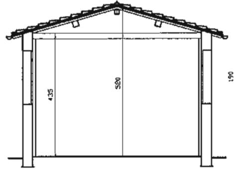
SEZIONE Y-Y invariato
